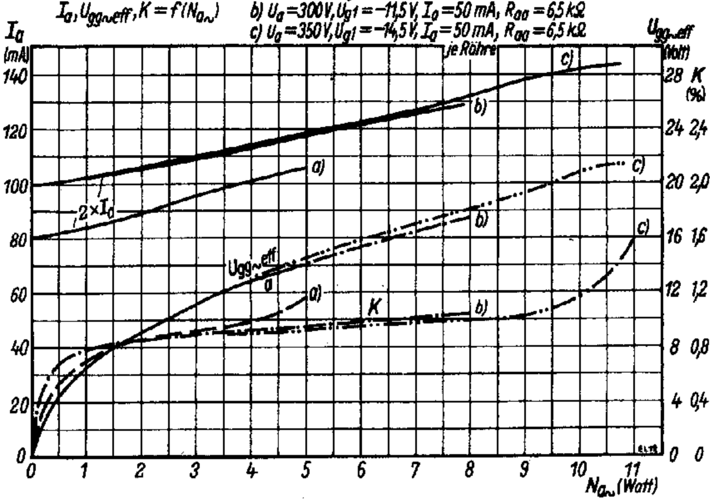
Kennlinienfeld 23
