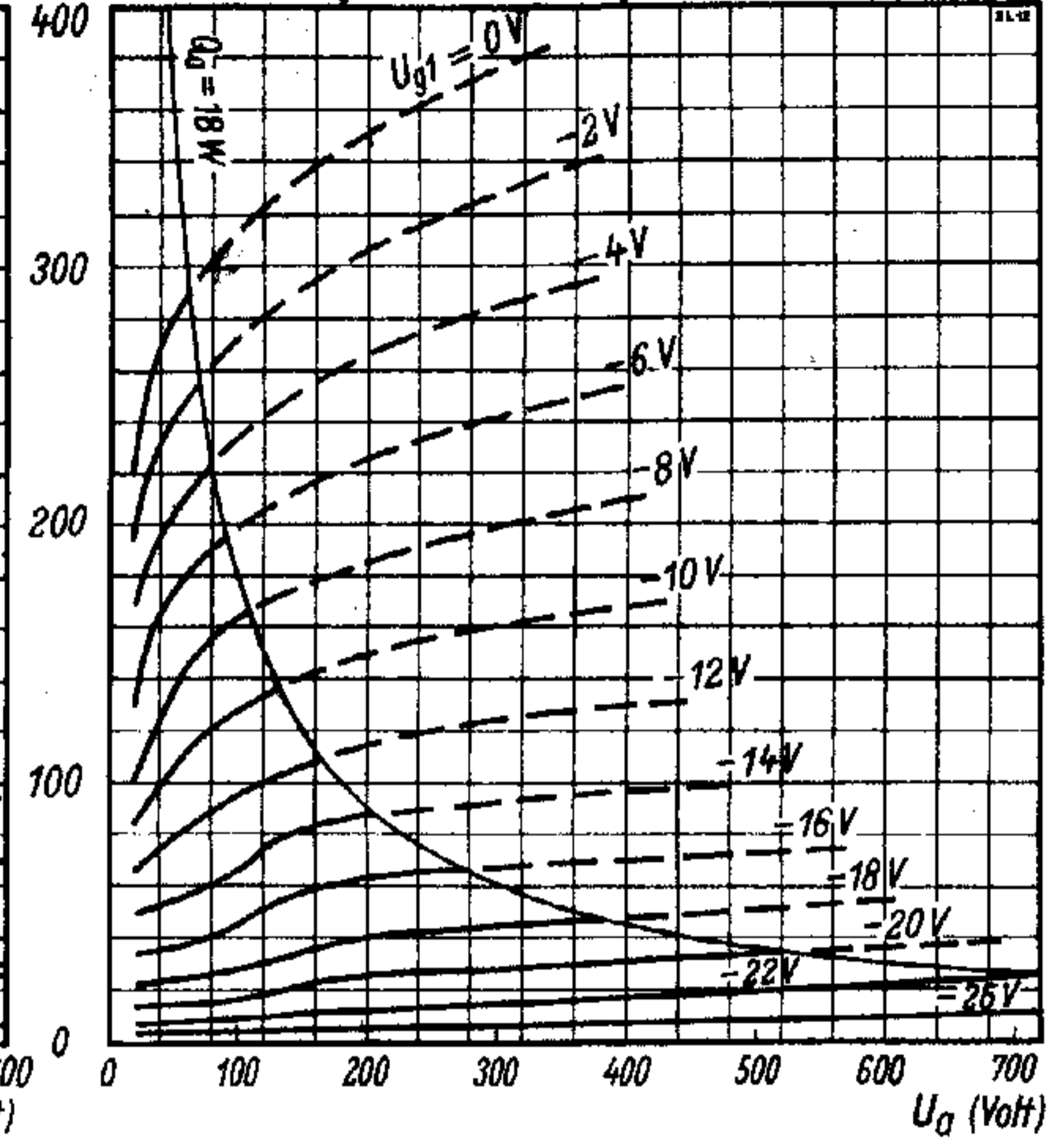
Kennlinienfeld 12 I_a = f(U_a)
