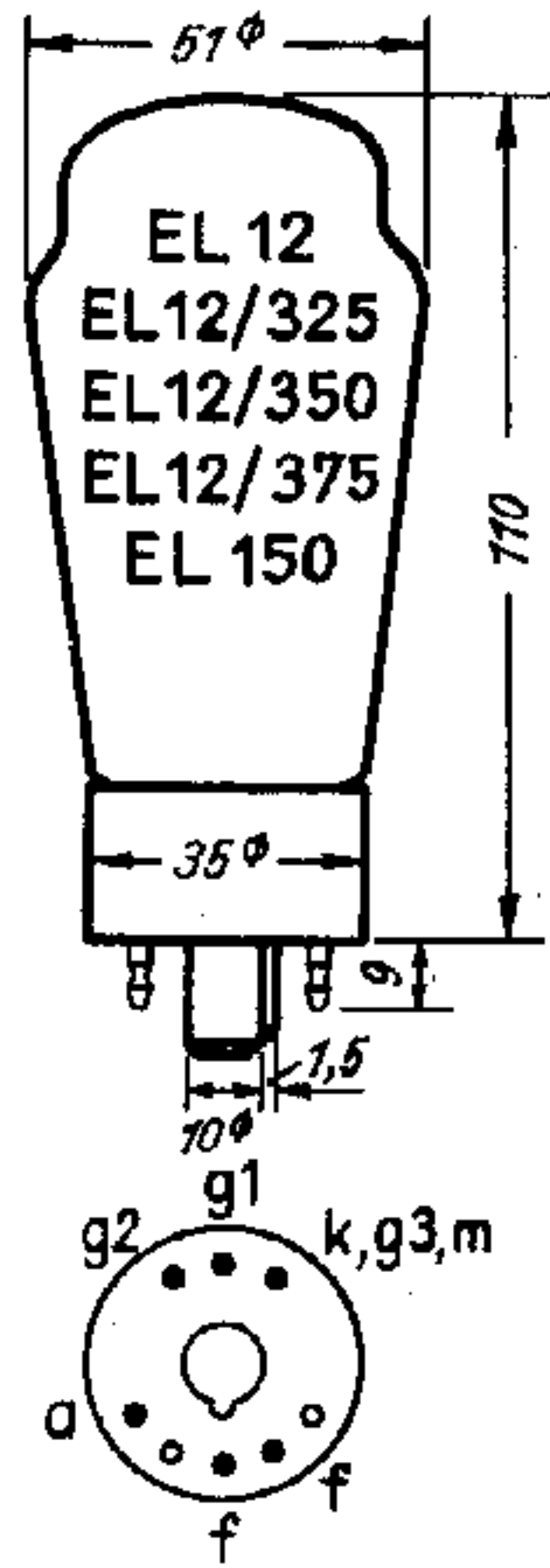
Sockel von unten gesehen
