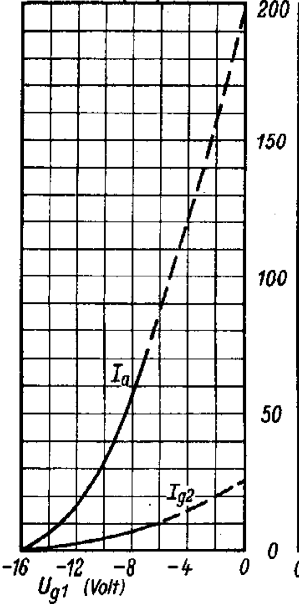
Kennlinienfeld 1 I_a, I_{g2} = f(U_{g1})
