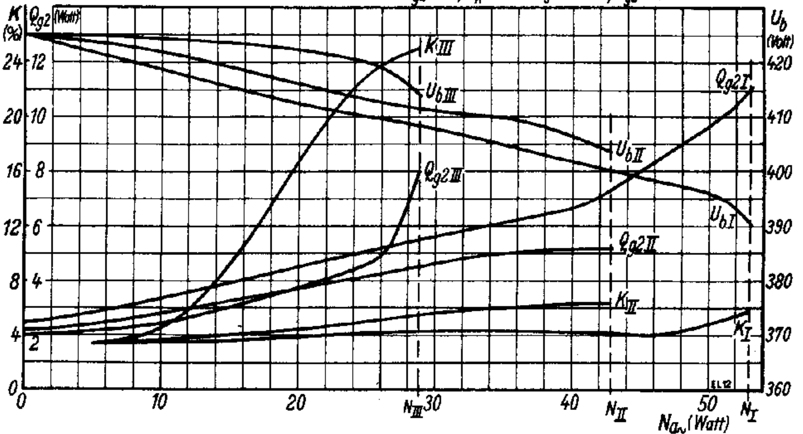
Kennlinienfeld 18 U_b, K, Q_{g2} = f(N_{av}) Alle Kurven reichen jeweils bis zum Gitterstromeinsatz Kurve I: U_{g1} und U_{g2} fest, R_{g2} u. R_k = 0 \Omega Kurve II: U_{g1} fest, R_{g2} = 4 \text{ k}\Omega je Röhre, R_k = 0 \Omega Kurve III: U_{g2} fest, R_k = 400 \Omega je Röhre, R_{g2} = 0 \Omega
