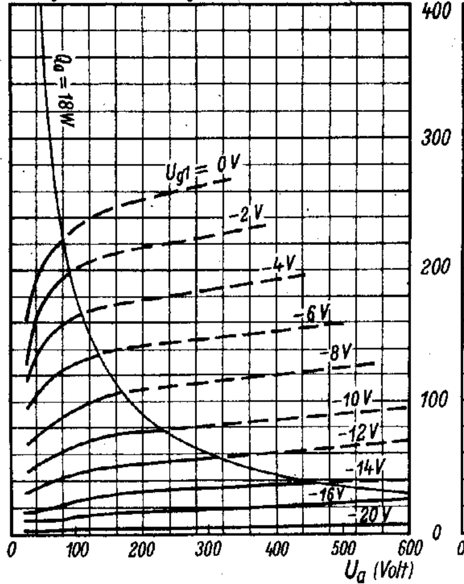
Kennlinienfeld 11 I_a = f(U_a)
