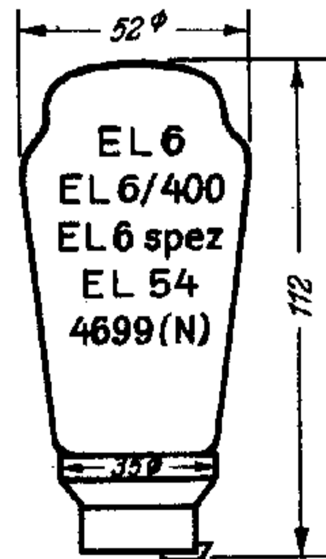
Kolbenabmessungen
