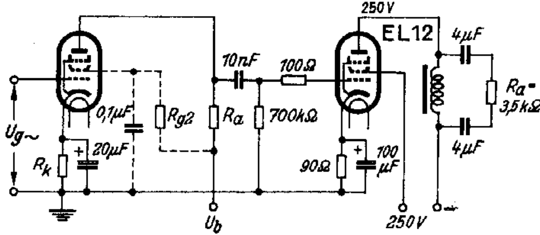
Schaltschema EL 12 + Vorstufe
