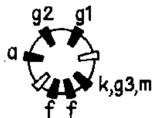
Socket von unten gesehen
