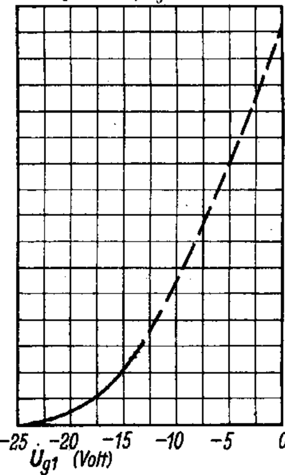
Kennlinienfeld 3 I_a = f(U_{g1})
